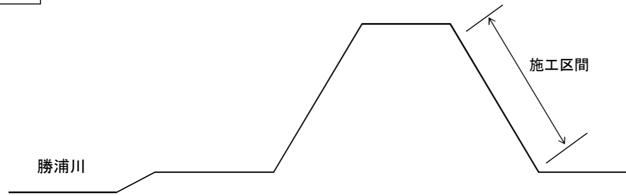
標準断面図
